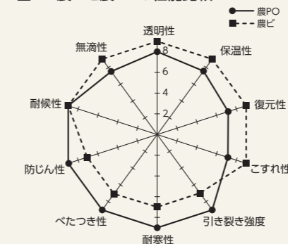
図2 農ビと農POの性能比較
